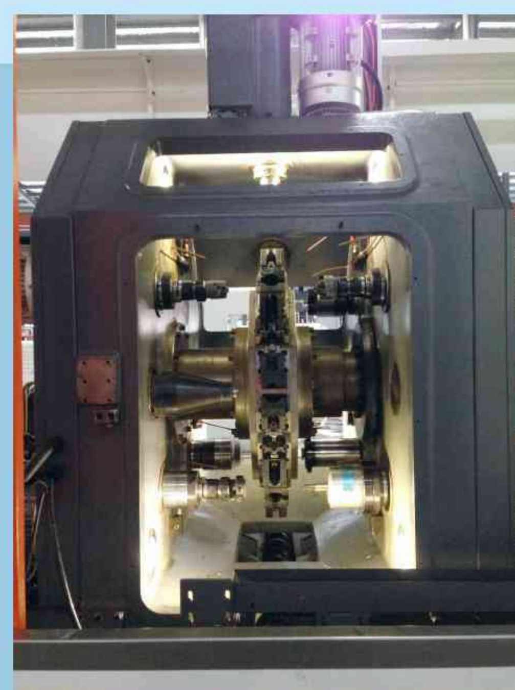
鼓轮式多主轴 钻车复合机床
